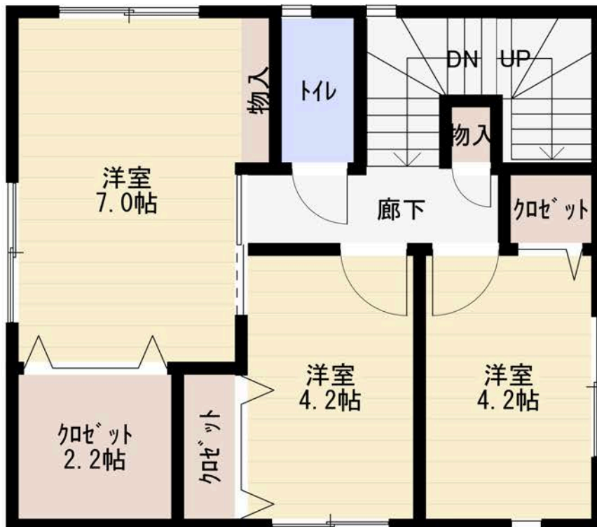
2階 縮尺 1/50
